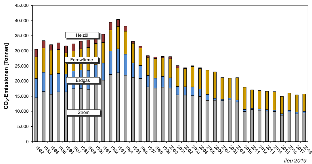
Abbildung 7: Entwicklung der CO 2 -Emissionen der Gebäude der Stadt Heidelberg (witterungskorrigierte Darstellung) *ab 2006 werden Erdgasverbräuche teilweise über die Wärmelieferung bilanziert, deshalb sind die Emissionen durch Erdgas in der Fernwärme enthalten.
