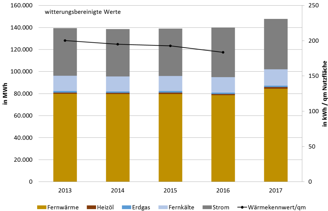
Abbildung 6: Entwicklung des Energieverbrauchs der Universität Heidelberg 2013 bis 2017 (witterungsbereinigt)
