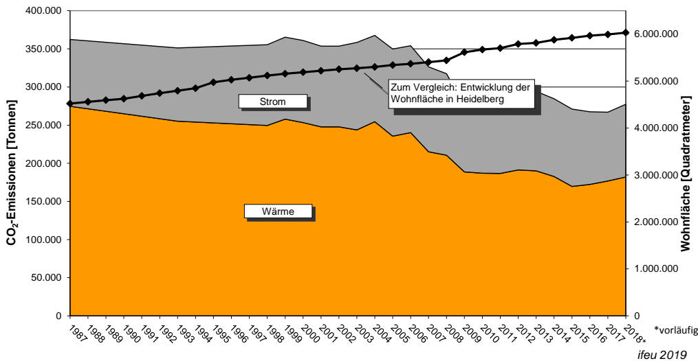
Abbildung 5: CO 2 -Emissionen der privaten Haushalte in Heidelberg 1987 bis 2018 nach Wärme und Strom (witterungskorrigierte Darstellung)
