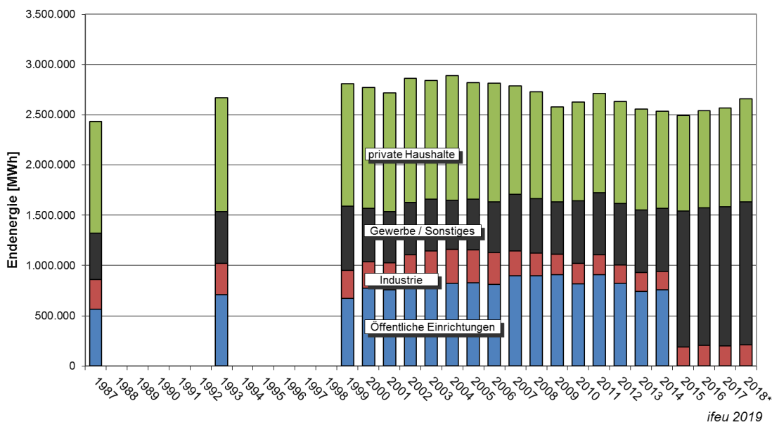
Abbildung 1: Entwicklung der stationären Endenergie in Heidelberg von 1987 bis 2018 nach Sektoren
