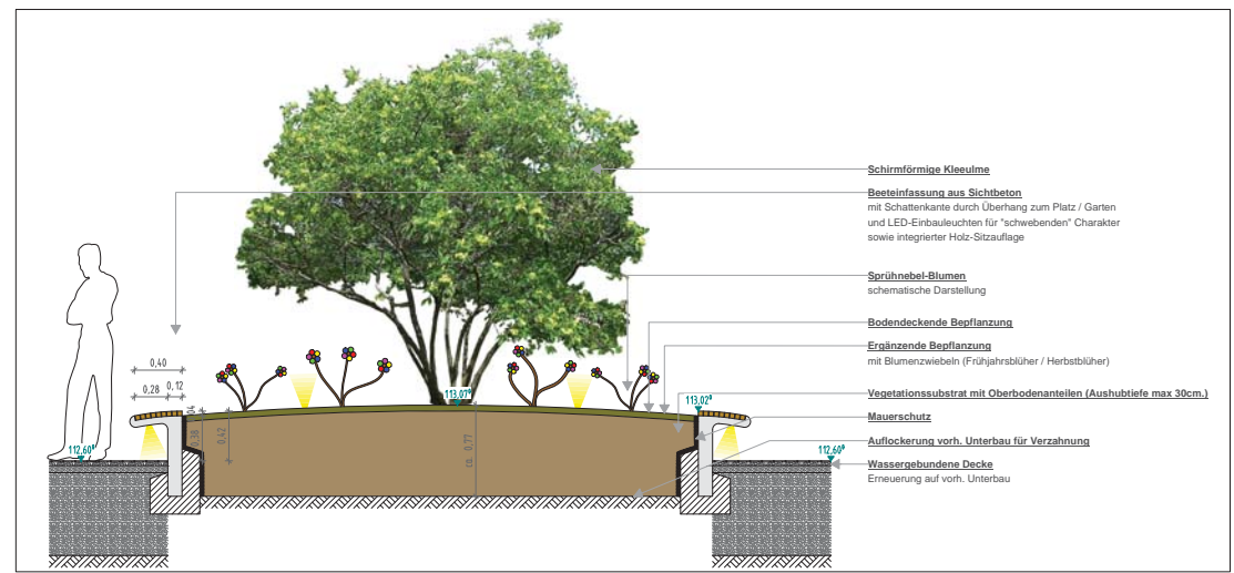
Schnitt durch Sitzelemente - M 1:25
