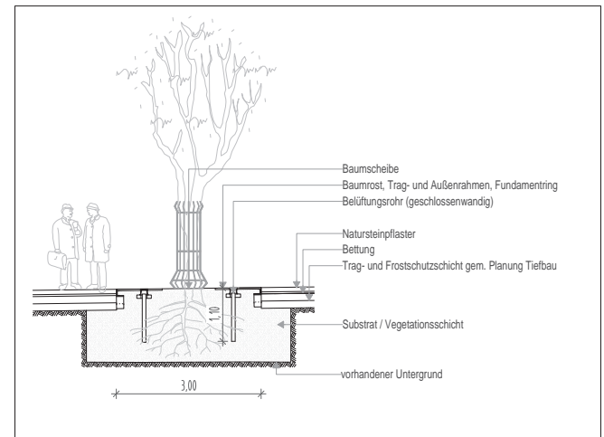
Schnitt Baumscheibe Theaterstraße - M 1:50
