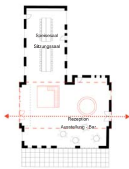
Grundrisse 1:200
